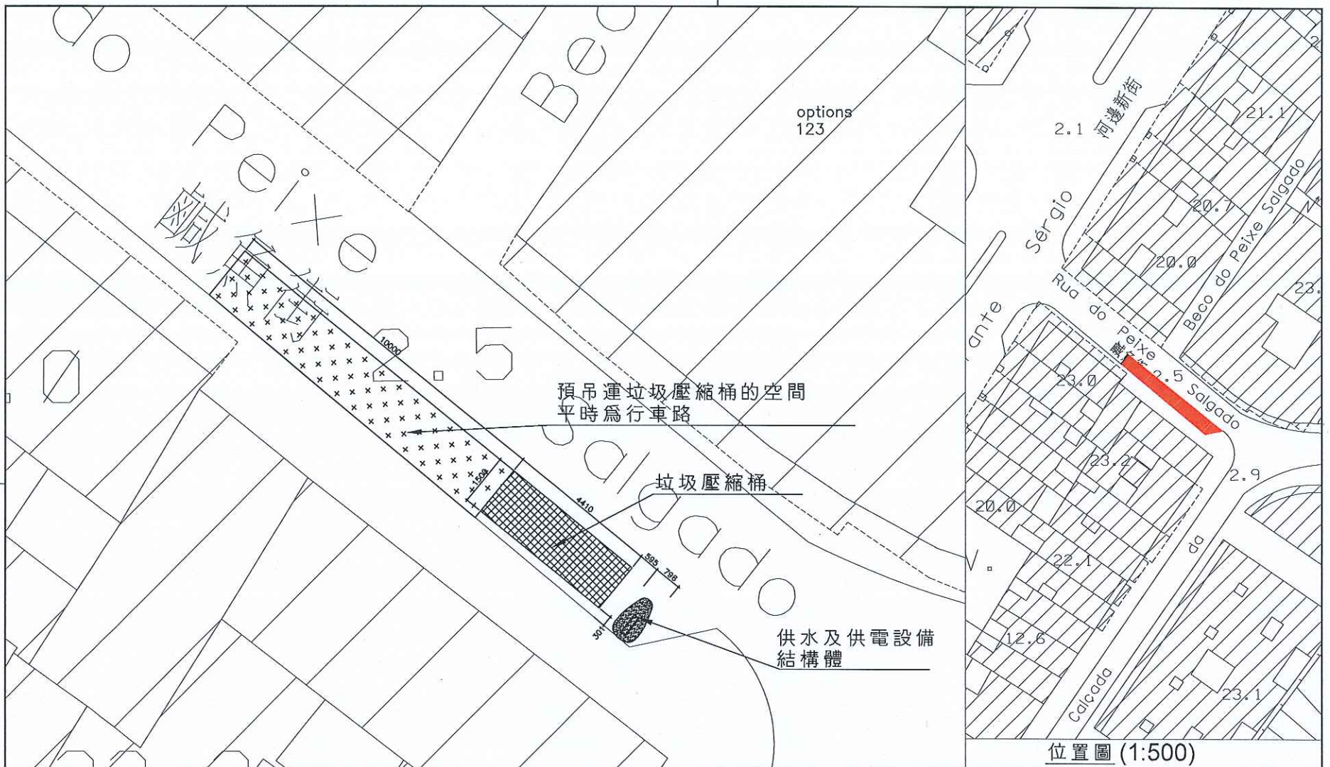
平面佈置圖 (1:100)
