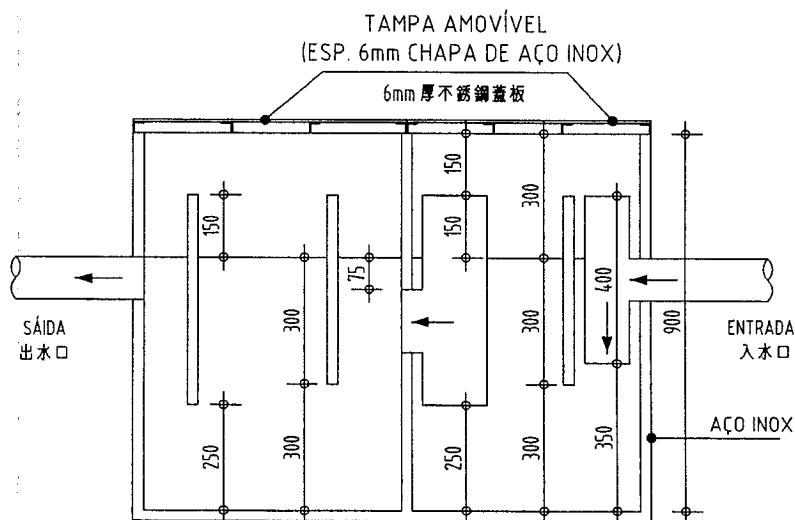
CORTE X-X 切面圖
