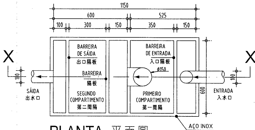
PLANTA 平面圖
