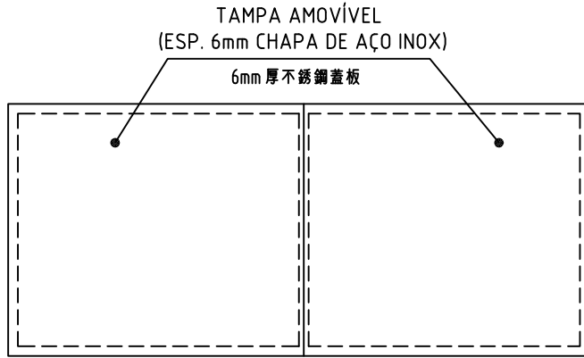
COBERTURA 頂視圖
