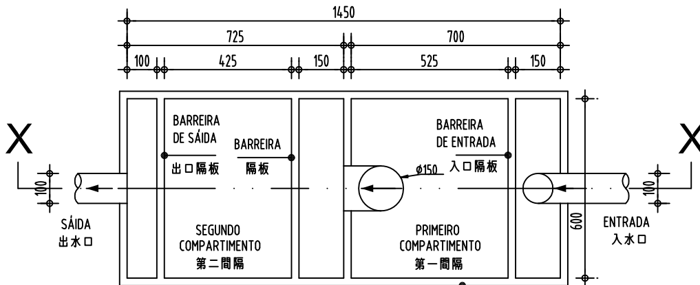
PLANTA 平面圖
