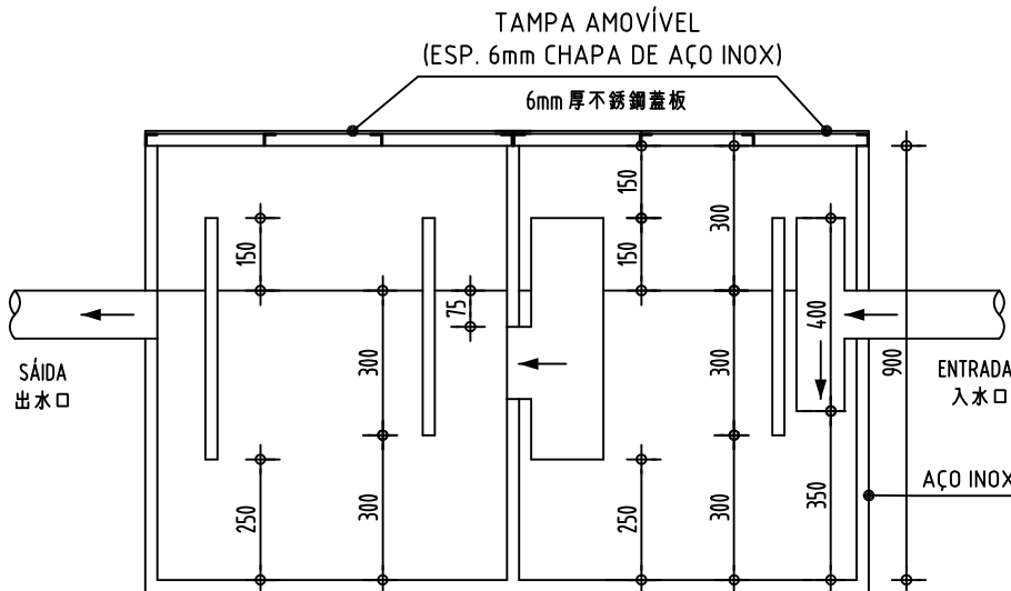
CORTE X-X 切面圖
