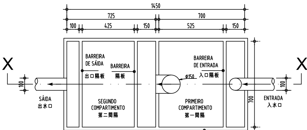
PLANTA 平面圖
