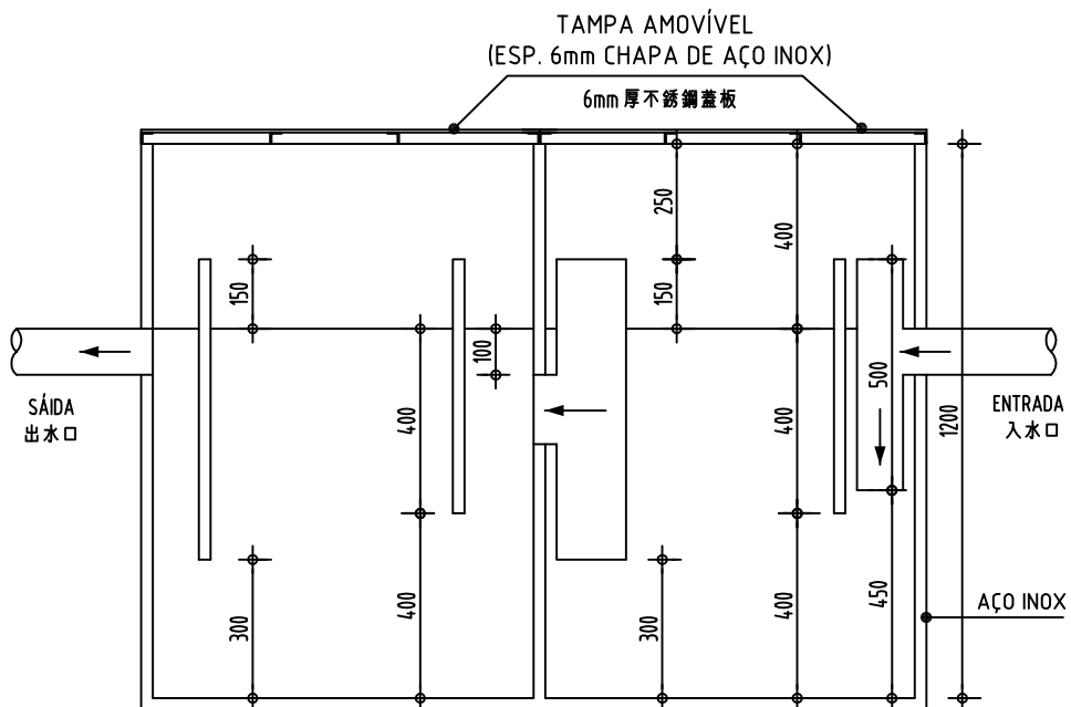
CORTE X-X 切面圖
