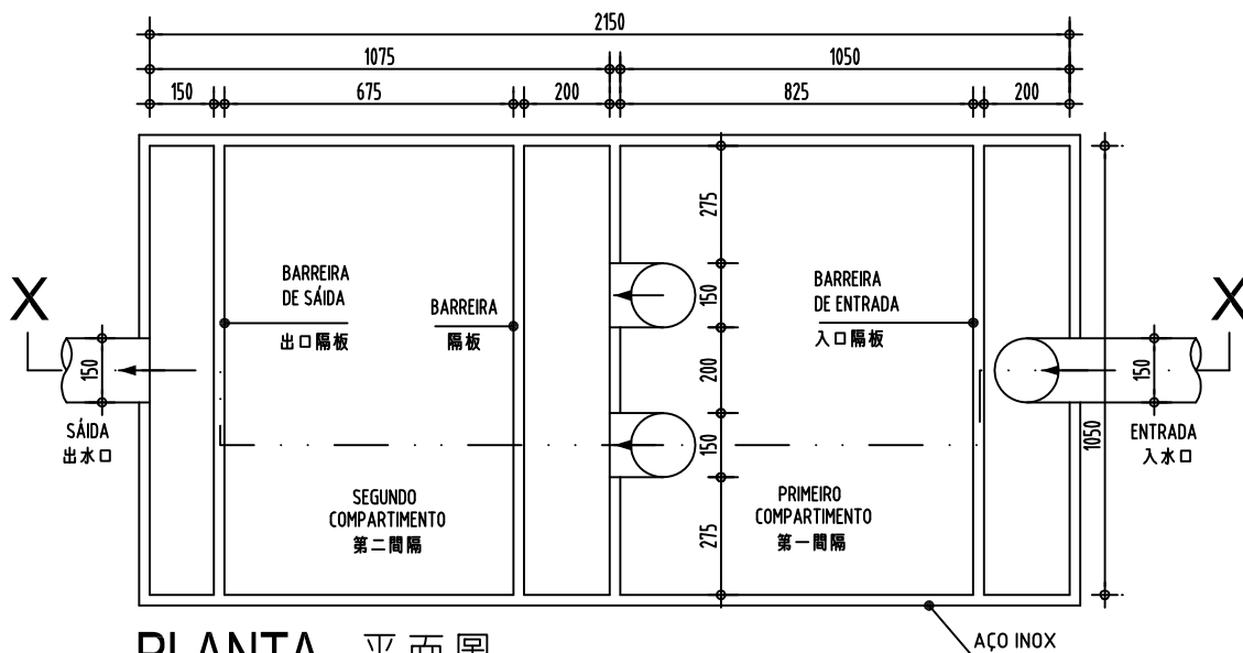
PLANTA 平面圖
