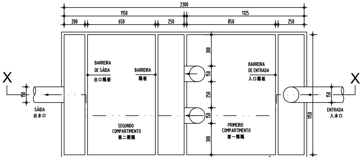
PLANTA 平面圖
