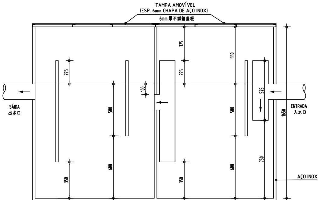
PLANTA 平面圖
