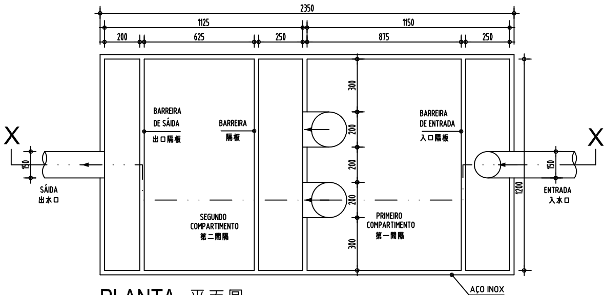
PLANTA 平面圖
