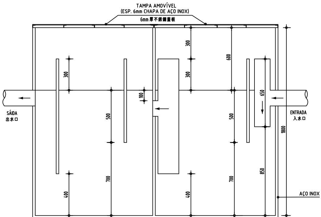
CORTE X-X 切面圖
