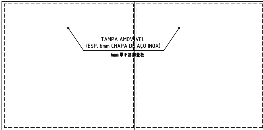
COBERTURA 頂視圖
