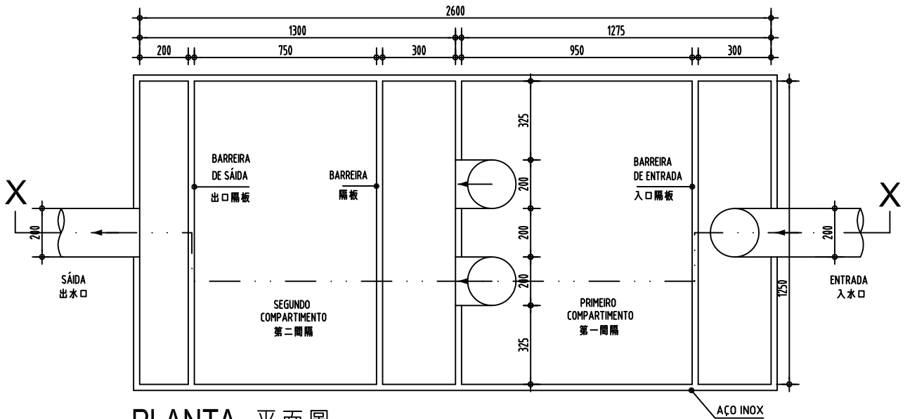
PLANTA 平面圖
