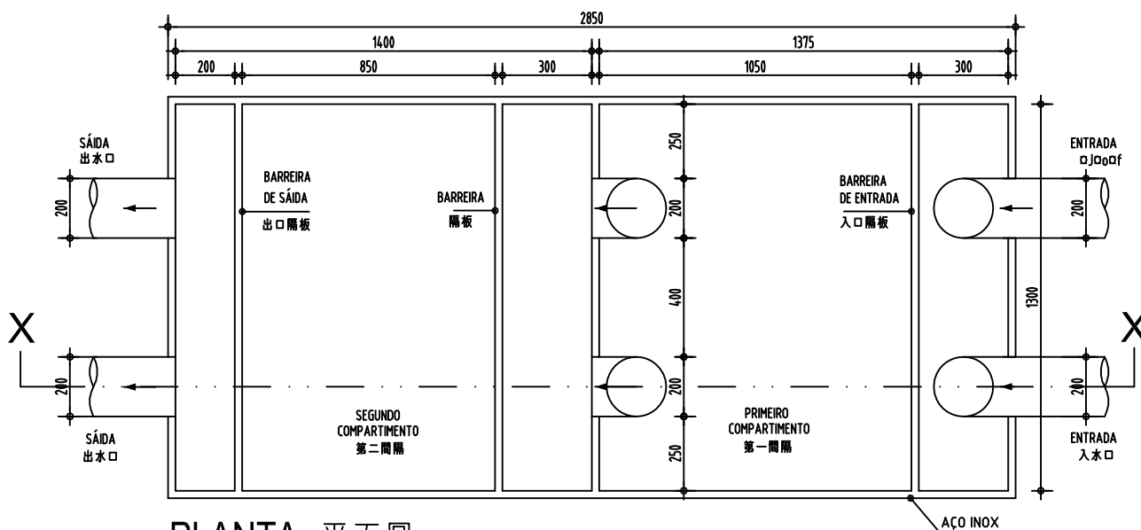
PLANTA 平面圖
